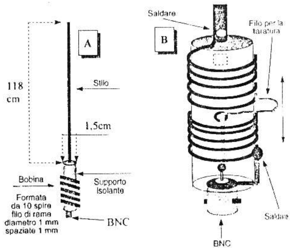
ANTENA 5/8 PARA VHF
