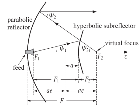
Fig. 17.11.1 Cassegrain dual-reflector antenna.
