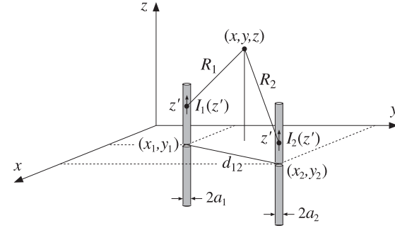
Fig. 21.3.1 Array of two linear antennas.
