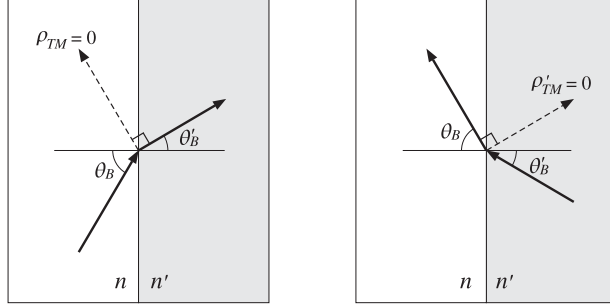
Fig. 6.6.1 Brewster angles.
