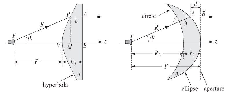
Fig. 17.12.1 Lens antennas.
