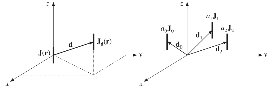
Fig. 18.2.1 Translated antennas.
