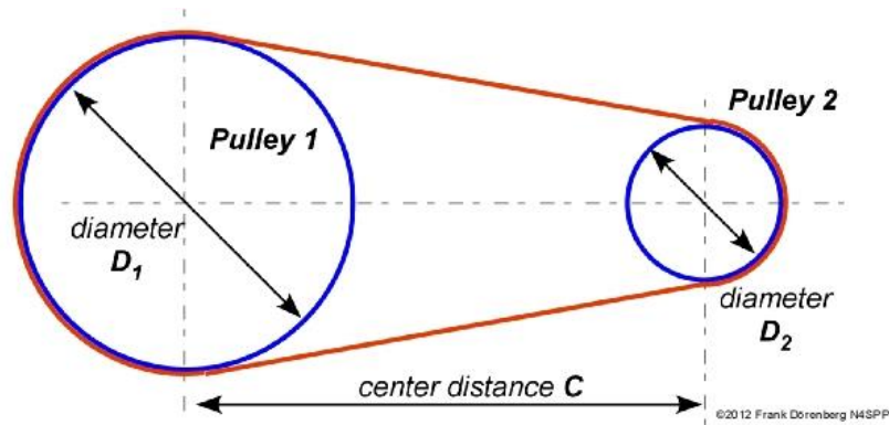
Fig. 98: Pulley configuration parameters
