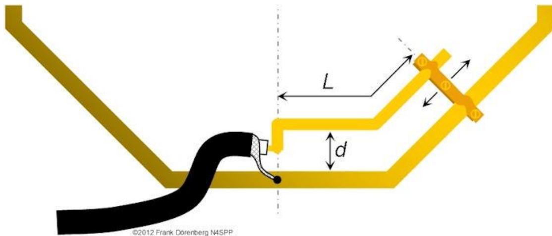
Fig. 33: Gamma Rod coupling
