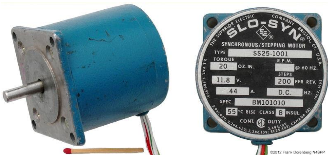
Fig. 89: An old Slo-Syn SS25-1001 motor
