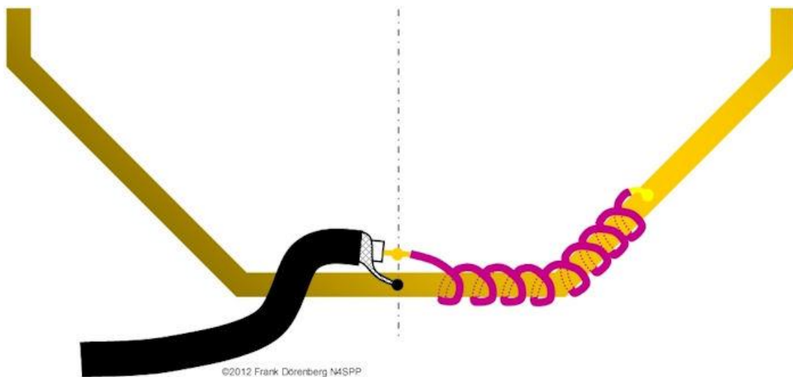
Fig. 37: Twisted-Gamma coupling
