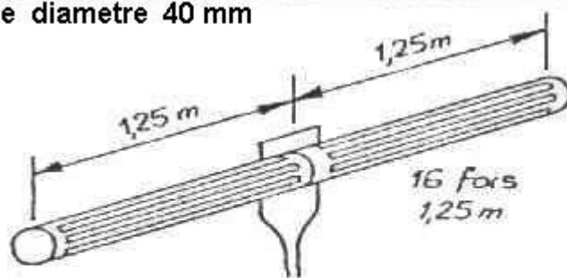
Antenne 14 MHz horizontale.
