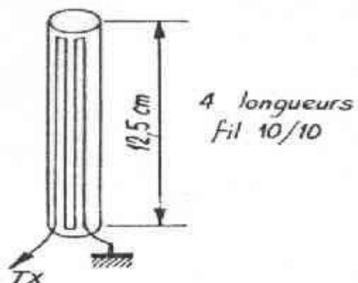
Antenne 144 MHz verticale.
